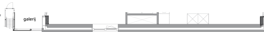
Zijgevel Type C15 huisnr. 13 plattegrond als type C11 ramen in zijgevel
