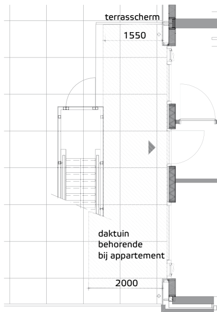
Daktuin Type C14 huisnr. 5 geen balkon maar daktuin geen galerij maar daktuin plattegrond als type C11
