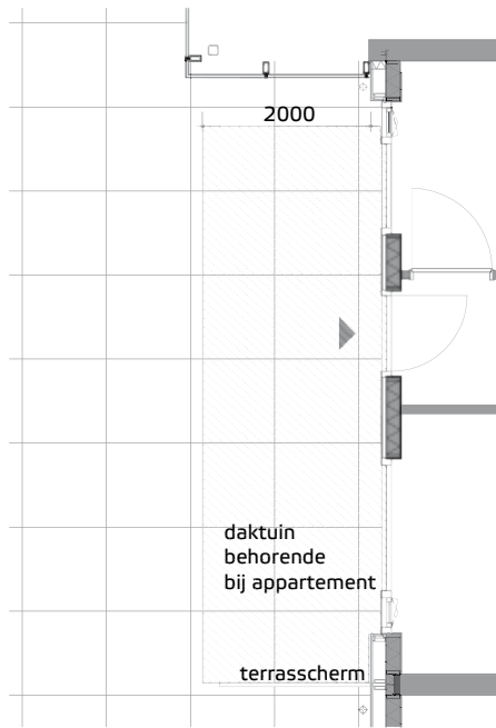
Daktuin Type C12 huisnr. 1+4 geen balkon maar daktuin geen galerij maar daktuin plattegrond als type C11
