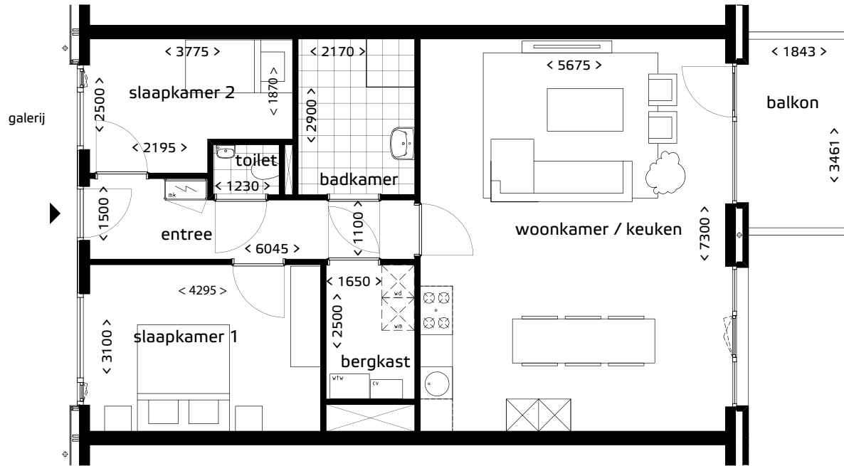
Type C11 huisnr. 8+10+12
